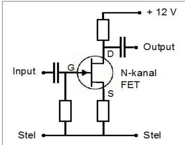
Forstærker i fælles source kobling Drain skal vende mod plus
